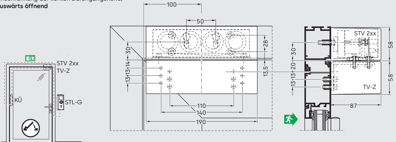
Montage bei flächenbündiger Tür über TV-Z an der Tür, ohne Einschränkung der lichten Durchgangshöhe, einwärts öffnend
