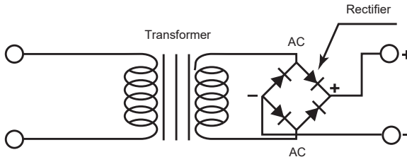
1 Amp Rectifier
