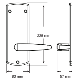
E2000 Interior
