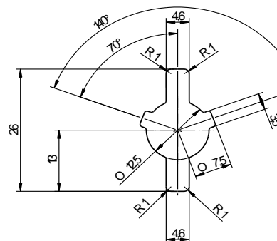
Skizze 2: Schlüsselträgerführung 86102
