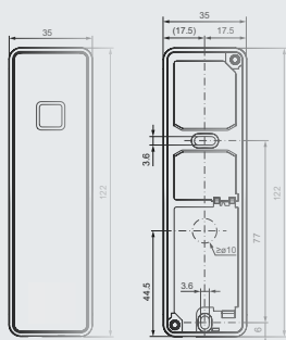
dormakaba läsare 9004 Front och bottenplatta
