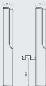
dormakaba läsare 9004, Sidvy med kabelutgång
