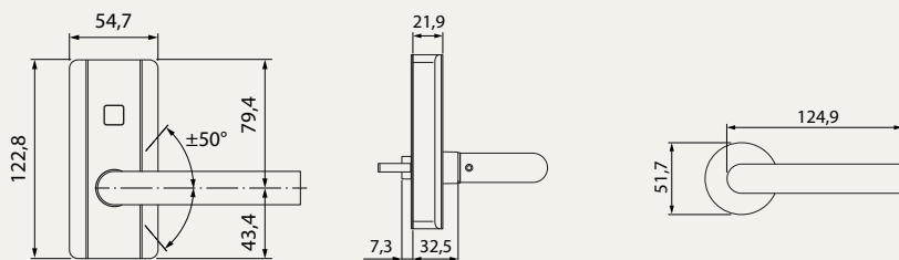
c-lever compact, exécution standard. Type 2725
