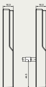
Lettore compatto dormakaba 91 04, vista laterale; versione IP66 con uscita del cavo.
