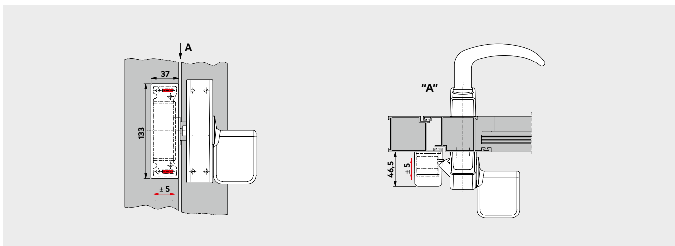
Esempio di applicazione di PHX 50 con Exit Pad su porta con profilo
