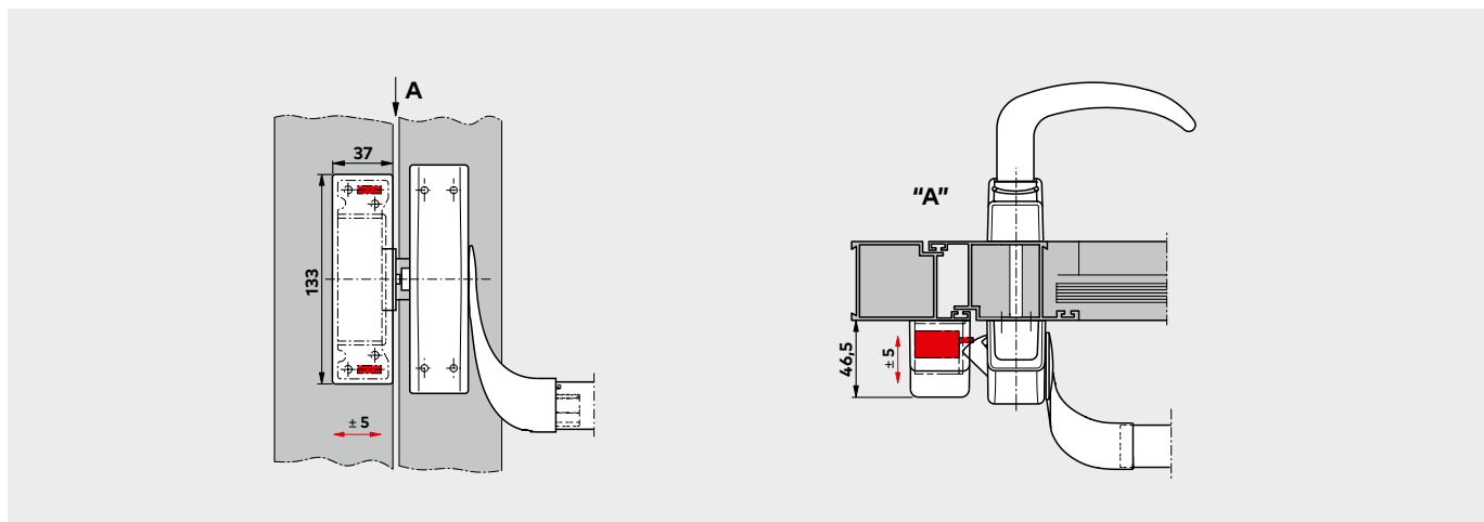
Esempio di applicazione di PHX 50 con PHA 2000 su porta con profilo
