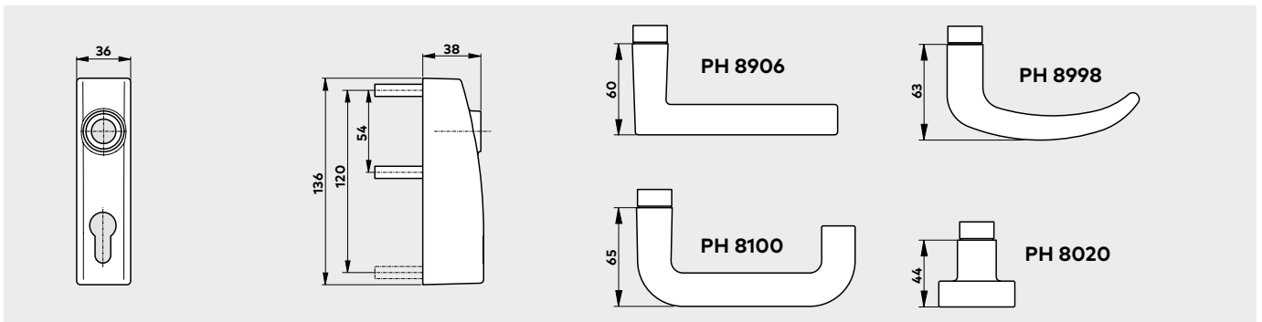
PHT 07 F – Base e modelli compatibili
