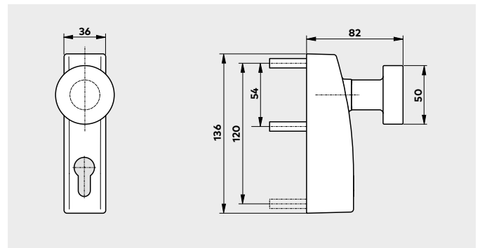
PHT 06 – Base con pomolo
