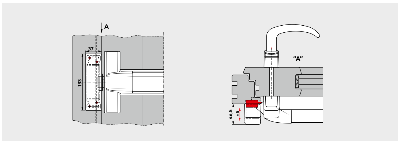
Esempio di applicazione di PHX 50 con PHB 3000 su porta con profilo
