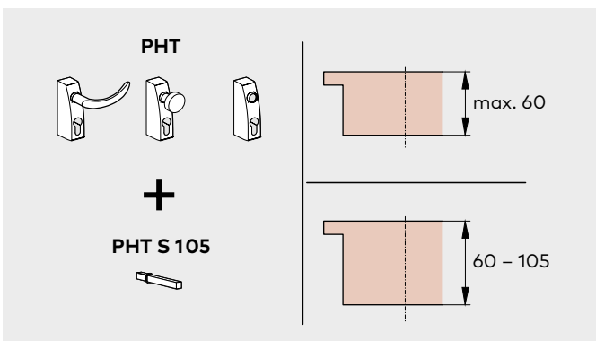
PHT 07 F – Base e modelli compatibili
