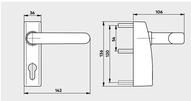
PHT 03, 05 F – Base con maniglia
