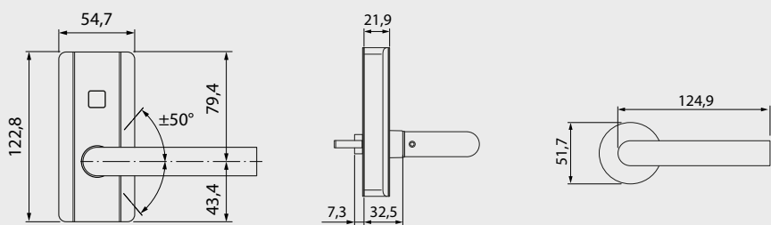
c-lever compact, versione standard Tipo 2725
