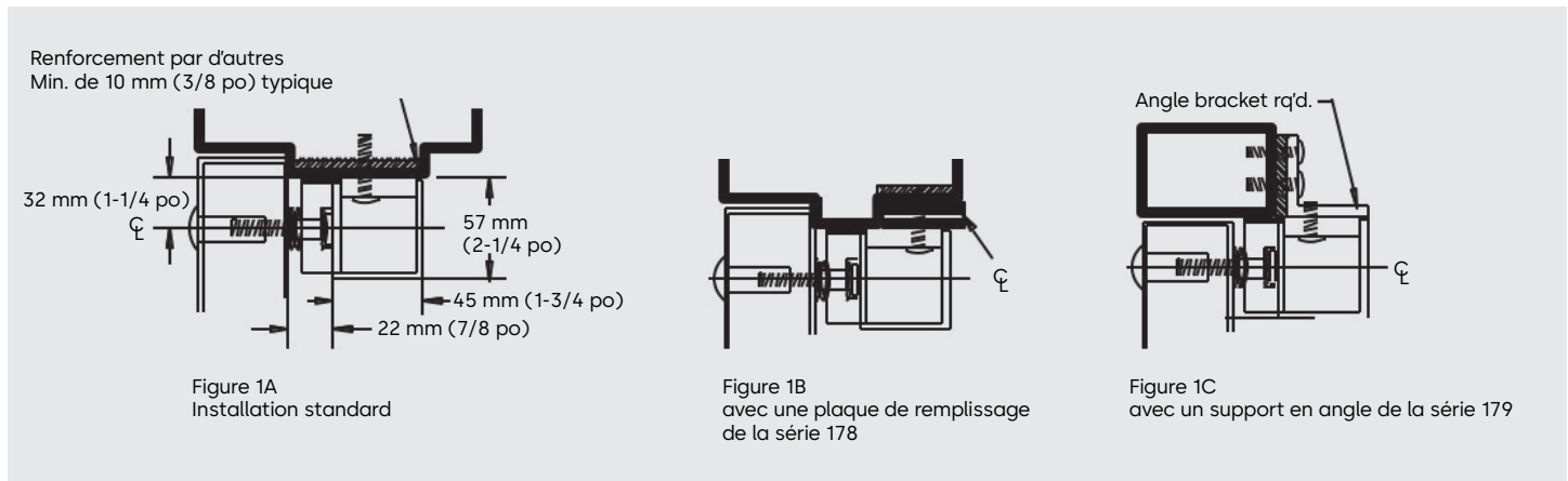
Figure 1 - Montage de la serrure magnétique sur le cadre
