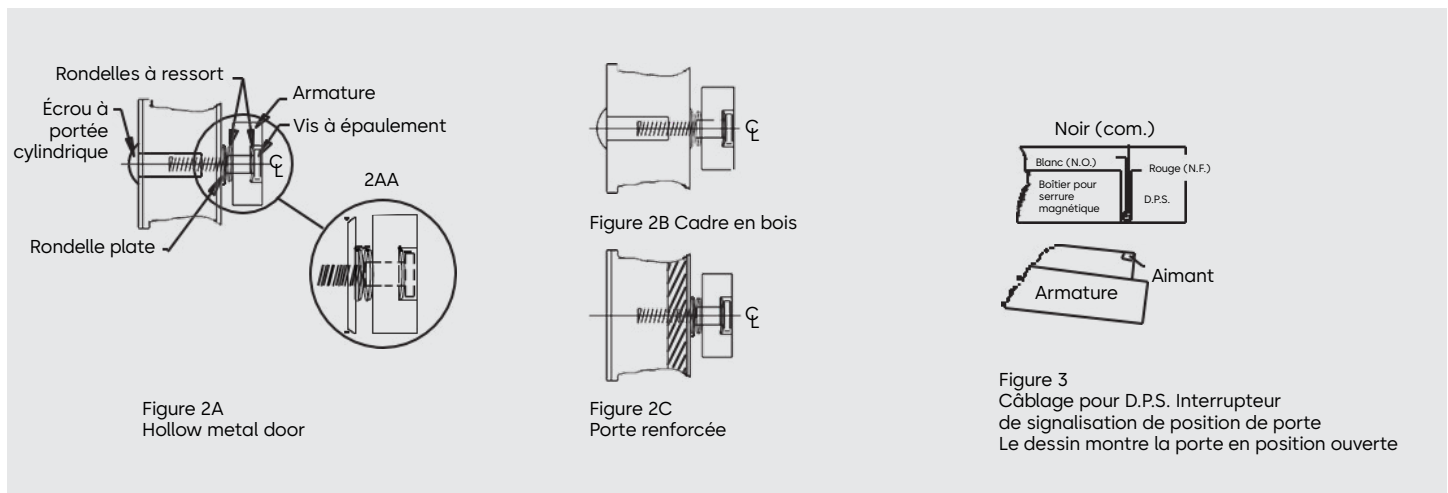
Figure 2 - Montage de l'armature sur la ou les portes
