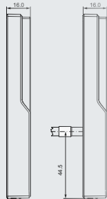
dormakaba Erfassungseinheit 90 04, Seitenansicht mit Kabelabgang
