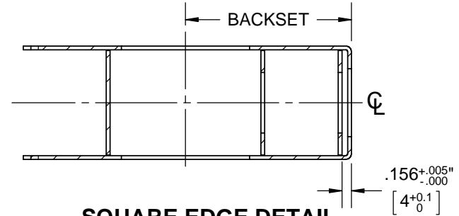
SQUARE EDGE DETAIL
