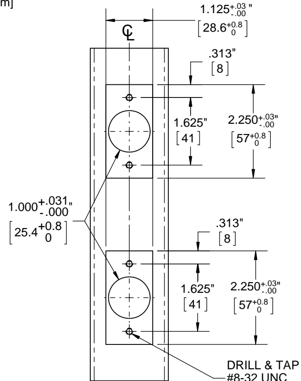
DOOR EDGE DETAIL
