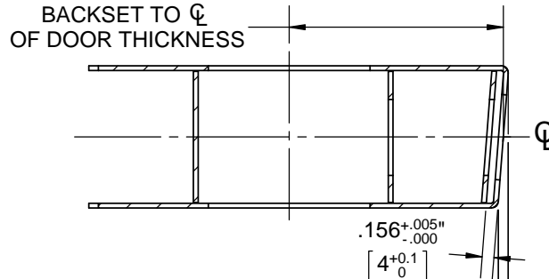
BEVELED EDGE DETAIL
