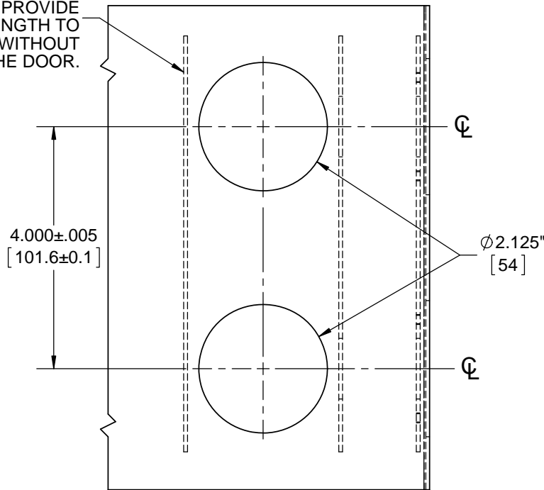
DOOR FACE DETAIL
