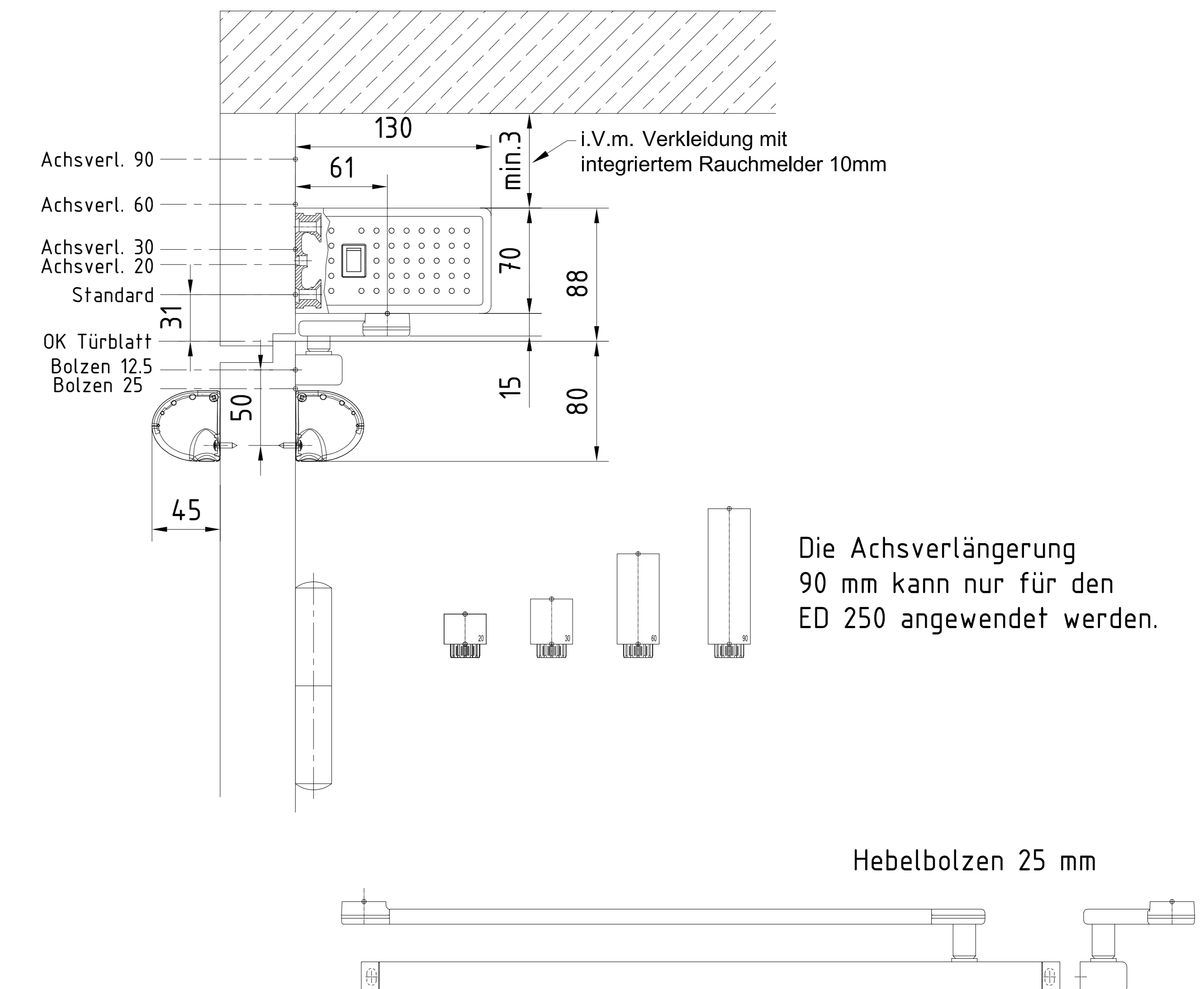
ziehend Gleitschiene mit ISR 4
