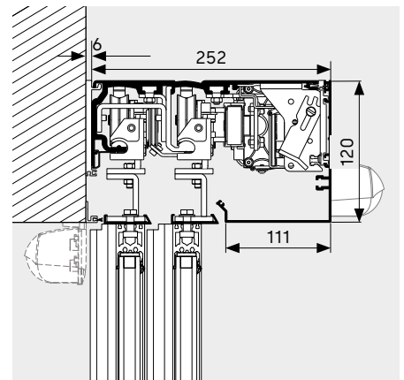
Skjematisk illustrasjon av dørtverrsnitt: veggmontert, drivhøyde 120 mm
