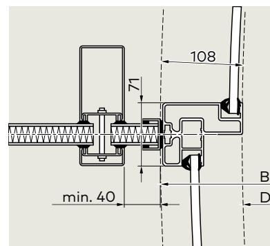
Versione con anta di chiusura notturna all'interno
