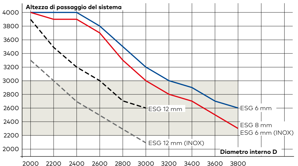
Altezza di passaggio del sistema tecnicamente possibile a seconda del diámetro interno D
