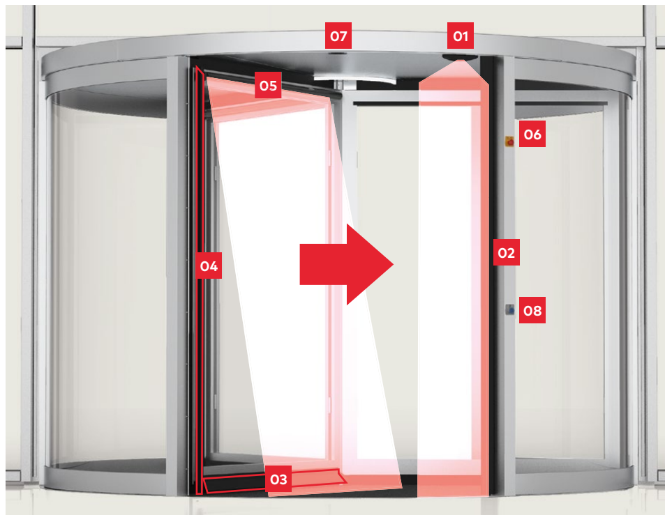
KTV A Funzionamento automatico
