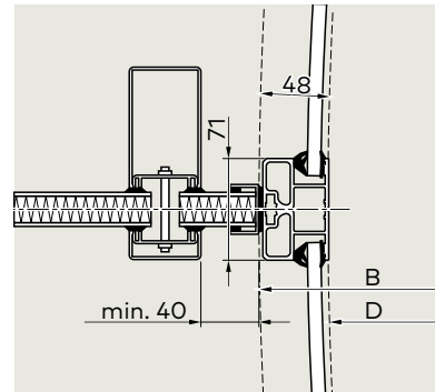
Versione senza chiusura notturna
