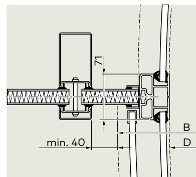
Versione con anta di chiusura notturna all'esterno
