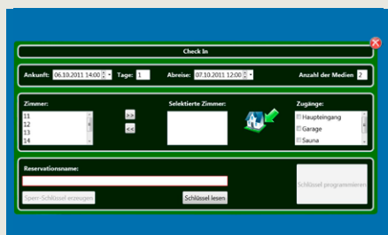
Modalità CheckIn: la programmazione delle tessere per gli ospiti avviene in modo specifico per determinate aree e determinati periodi di tempo.
